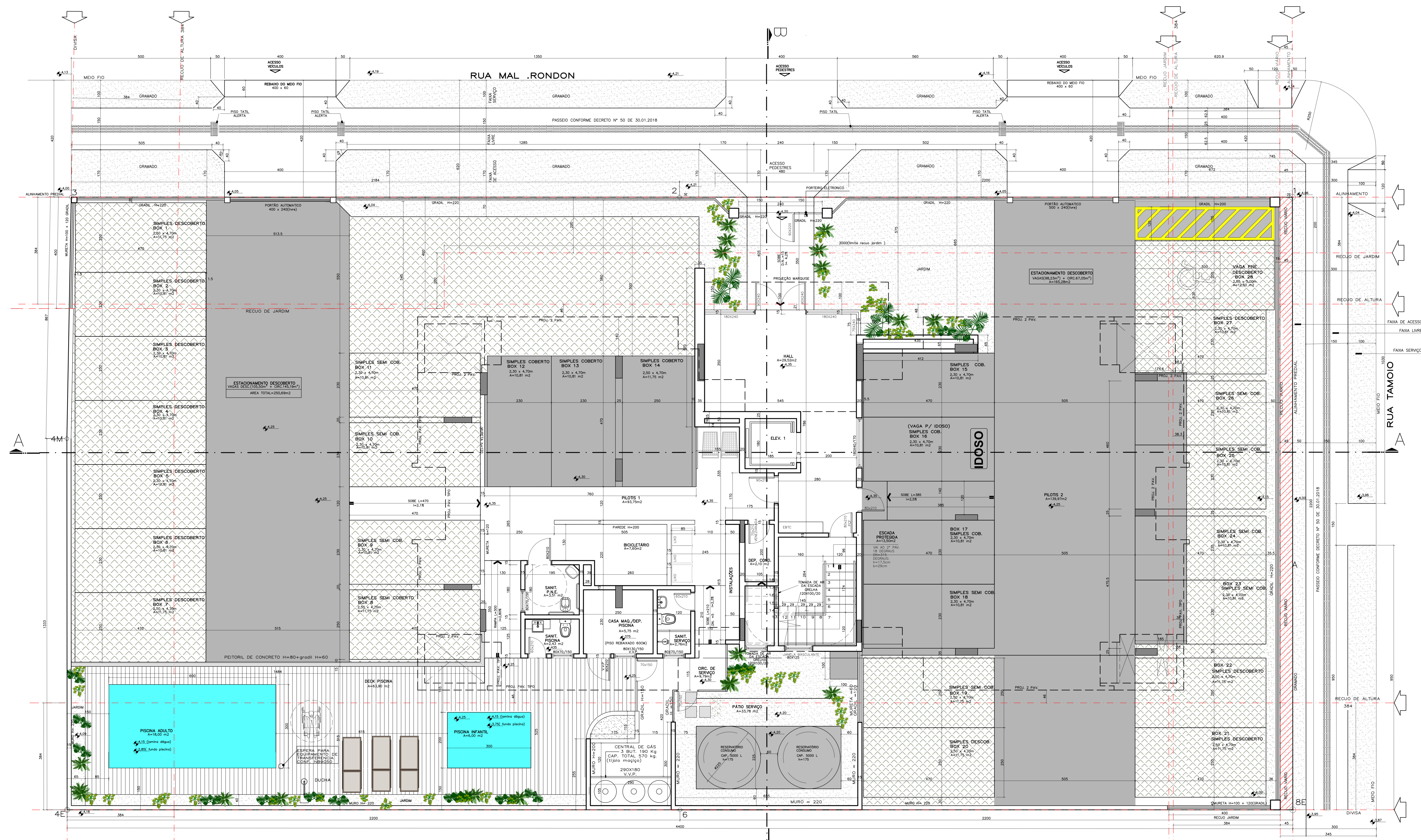
PLANTA BAIXA PAVIMENTO TÉRREO
