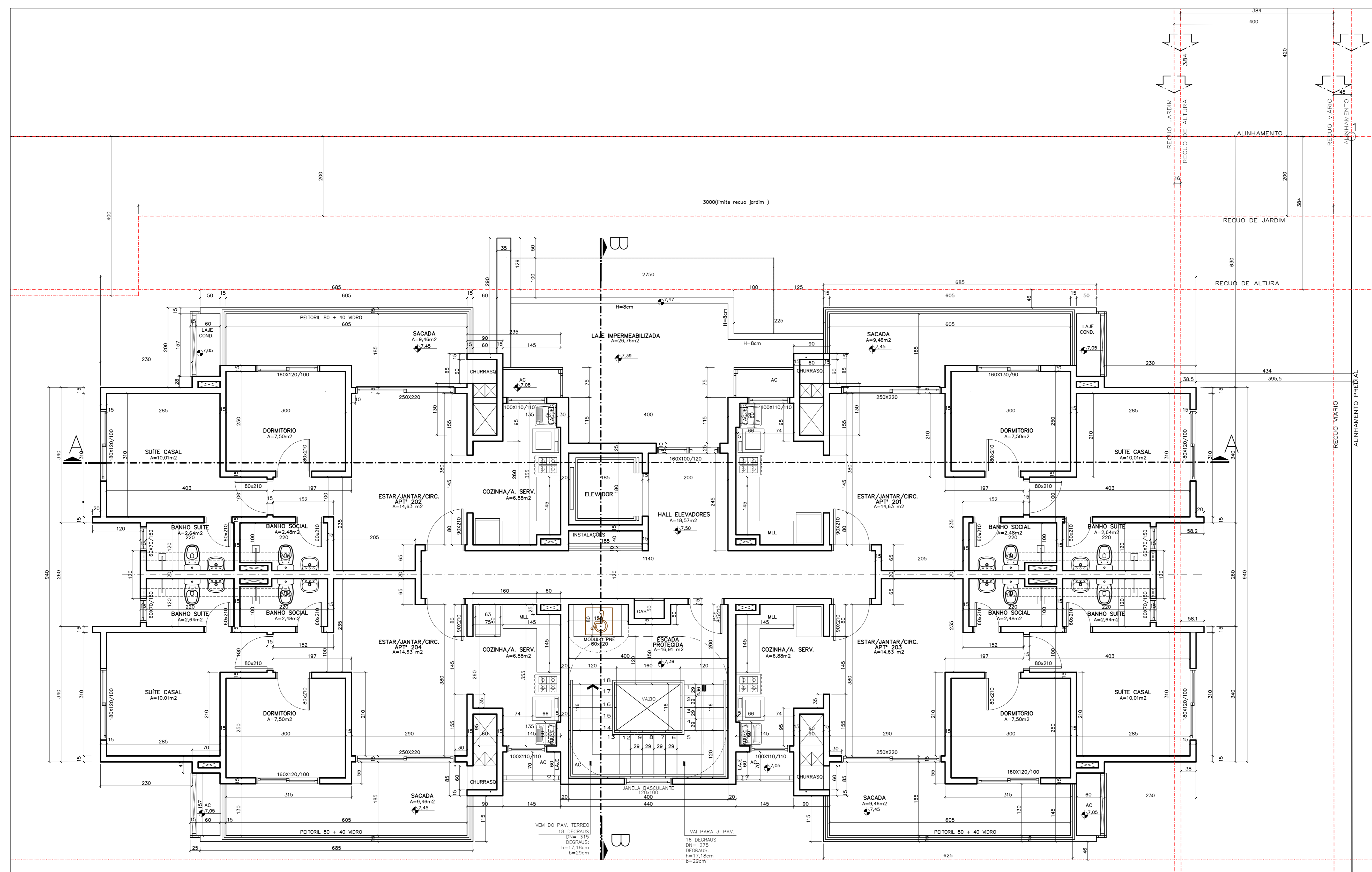
PLANTA BAIXA 2 - PAV. ESCALA 1:50
