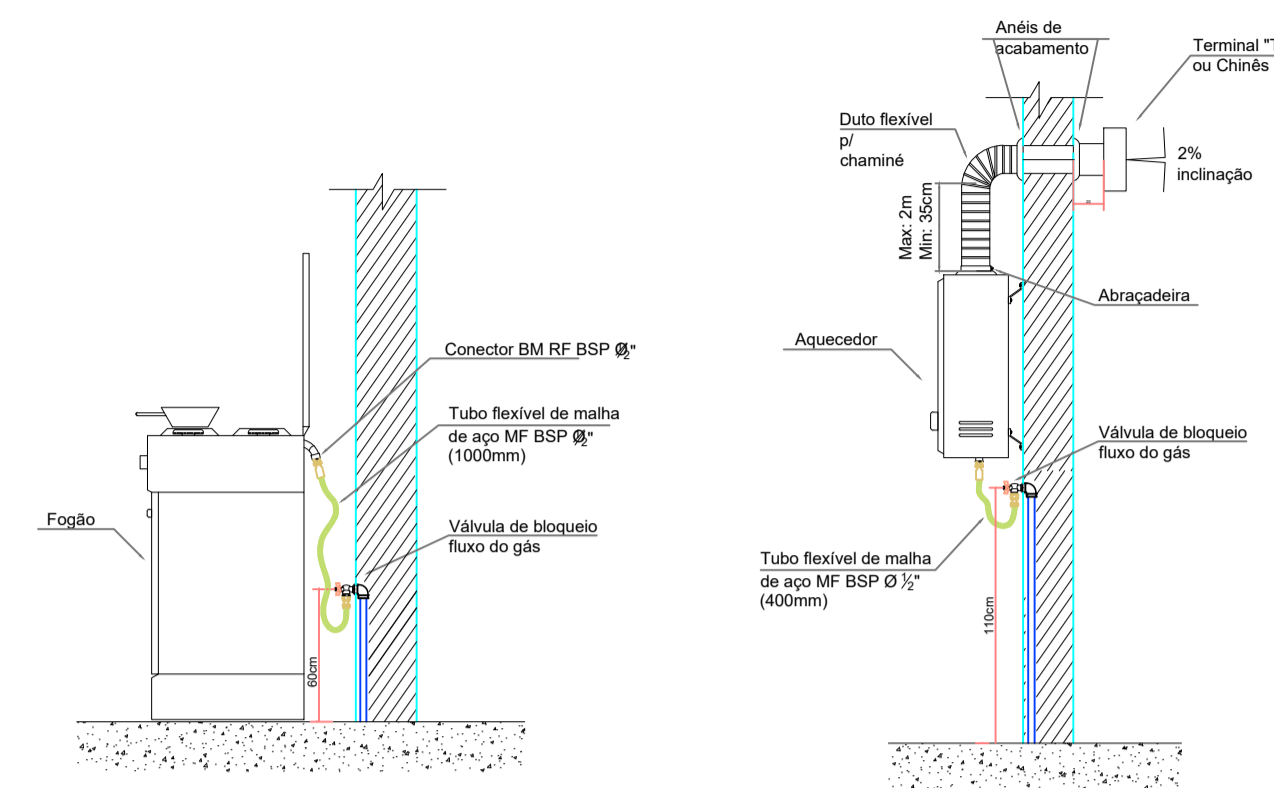
ESQUEMÁTICO PTOS DE CONSUMO FOGÃO e AQUECEDOR S/Esc.
